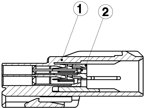
SEC. A-A
