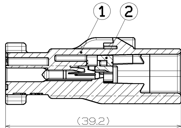
SEC. A-A
