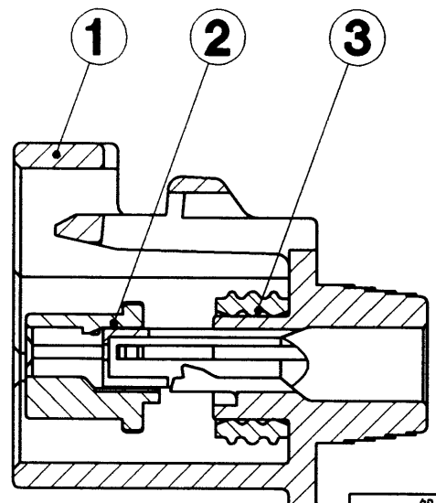
SEC. A-A
