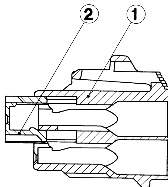
SEC. A-A
