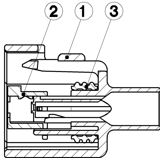
SEC. A-A
