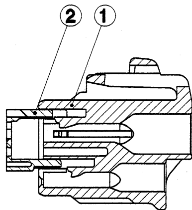
SEC. A-A
