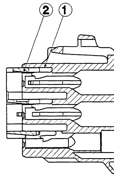
SEC. A-A
