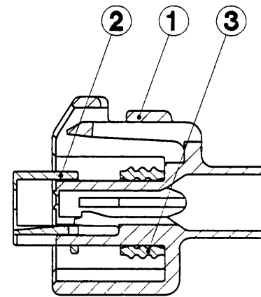
SEC. A-A
