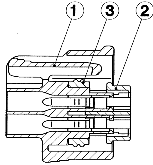
SEC. A-A
