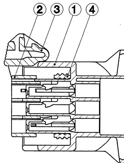
SEC. A-A
