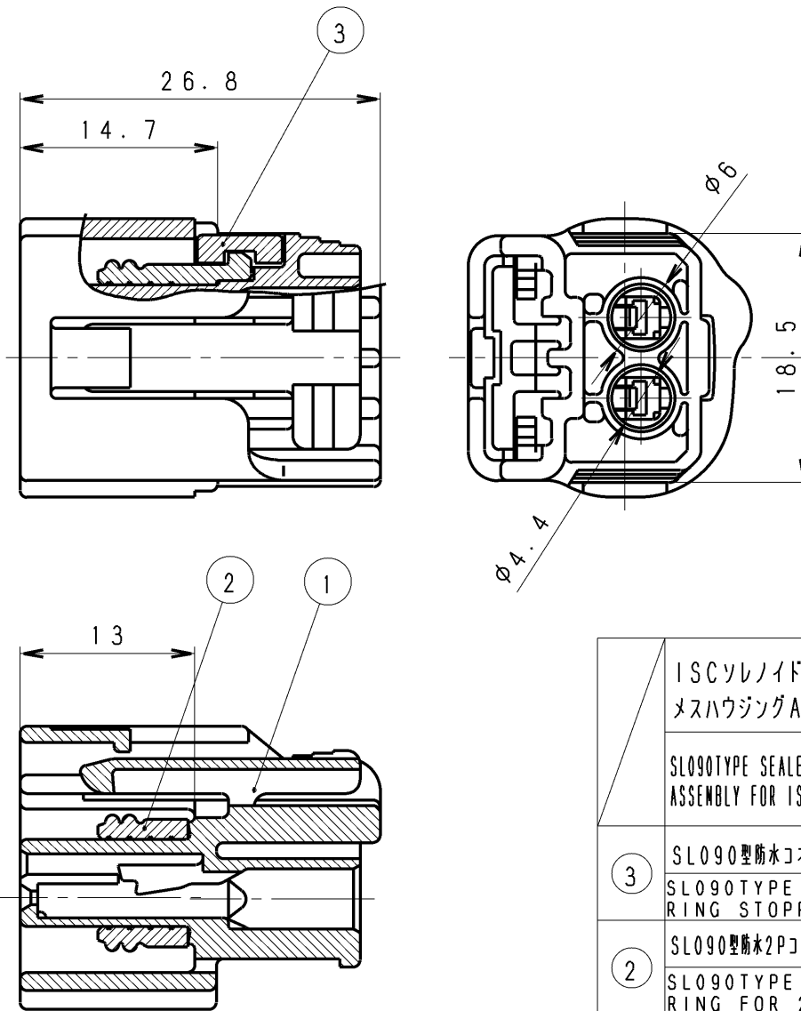
SECTION A-A
