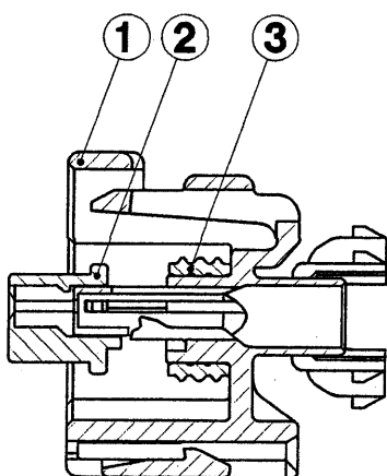
SEC. A-A
