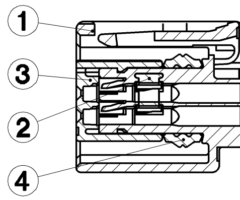
SEC. A-A
