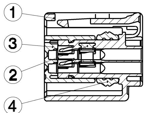
SEC. A- A
