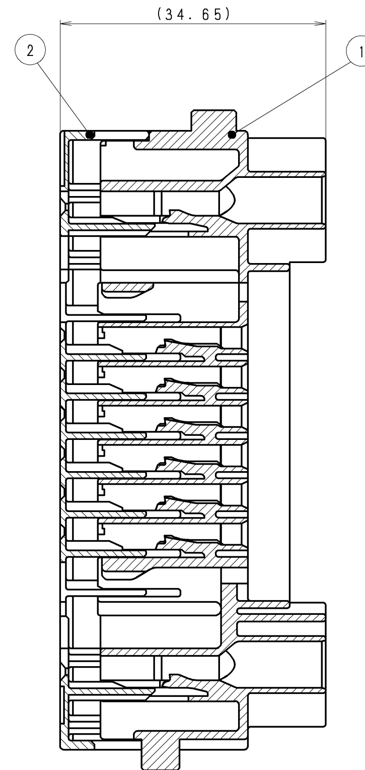
SECTION A-A
