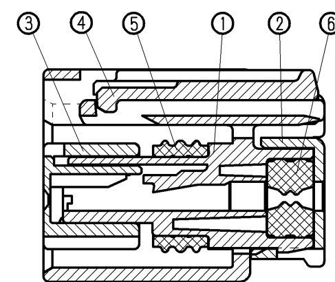
SEC. A- A
