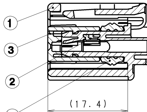
SEC. A-A
