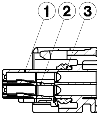
SEC. A-A
