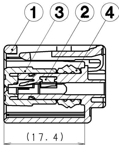
SEC. A-A
