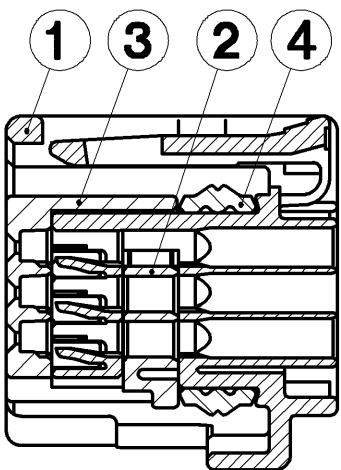
SEC. A-A
