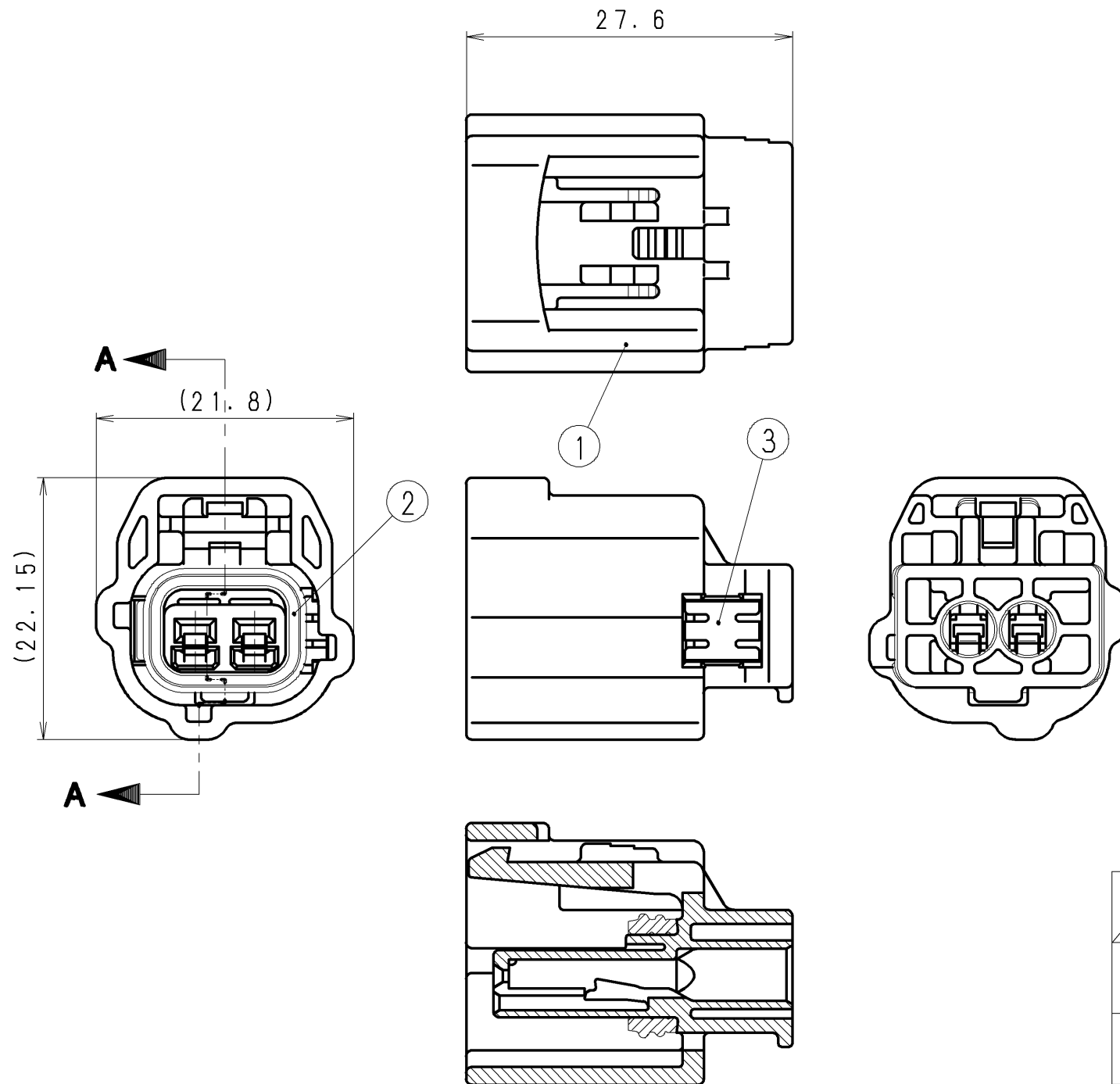
SECTION A-A
