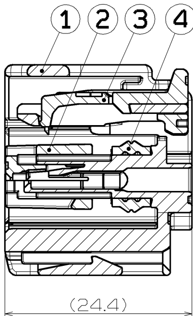
SEC. A-A
