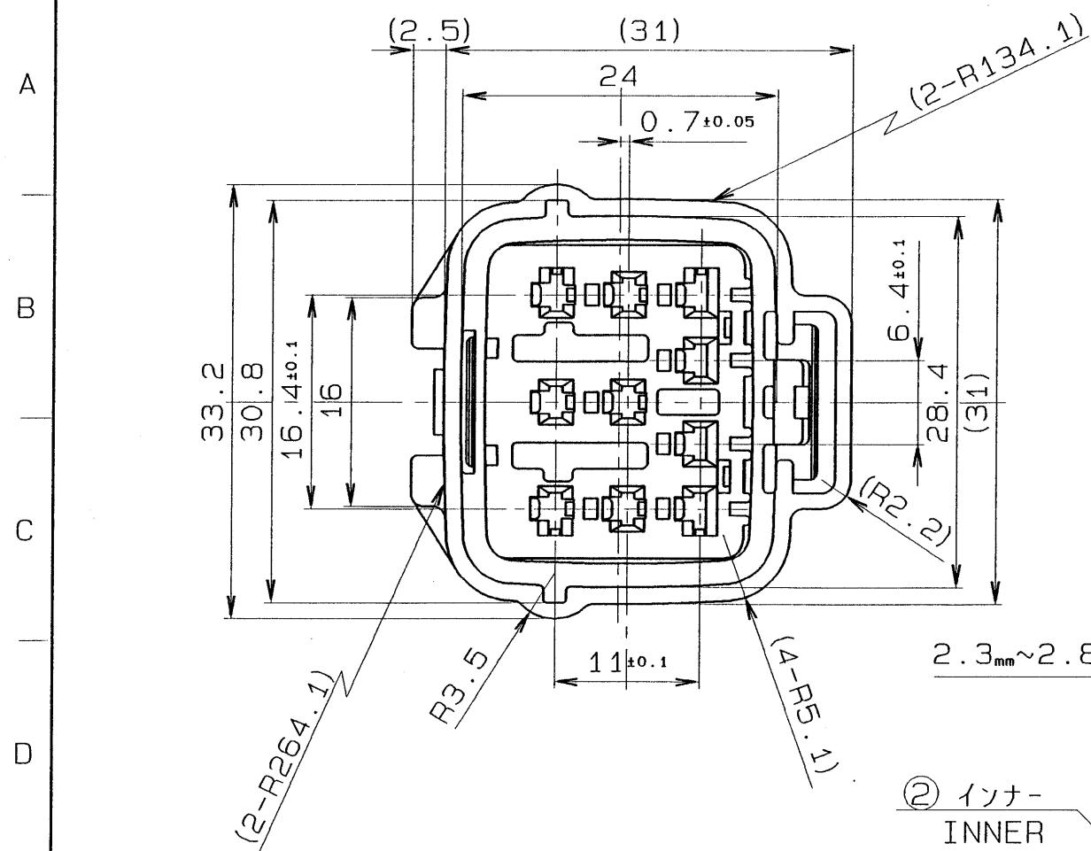
<ハウジングASSY品 & ASSY構成部品一覧表> <HOUSING ASSEMBLY & ASSEMBLED PARTS TABLE>
