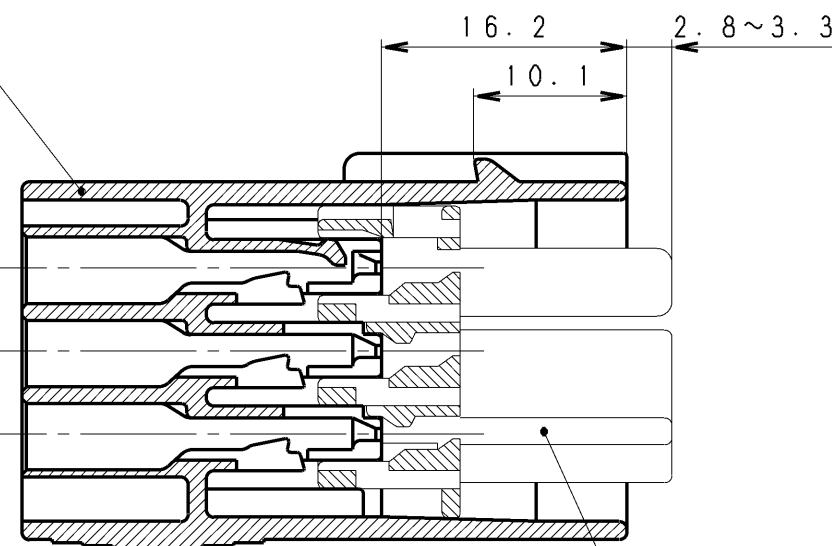
リテーナ (RETAINER) MATERIAL : PBT
