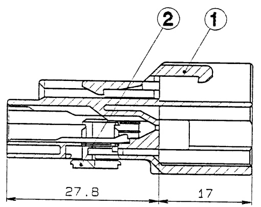
SEC. A-A
