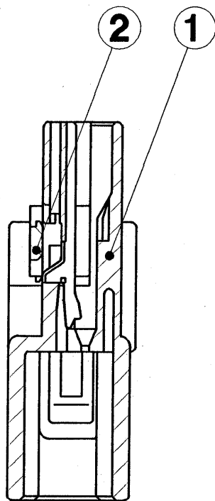
SEC. A-A
