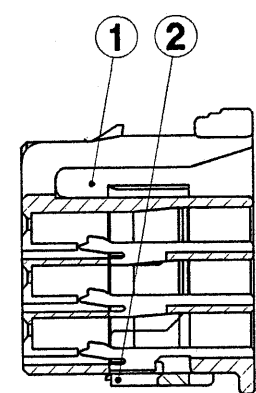
SEC. A-A
