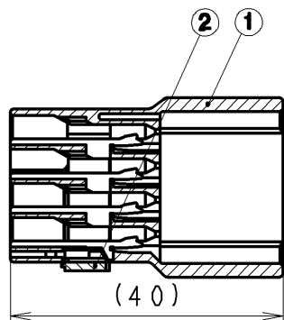
SEC. A-A
