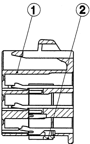
SEC. A-A
