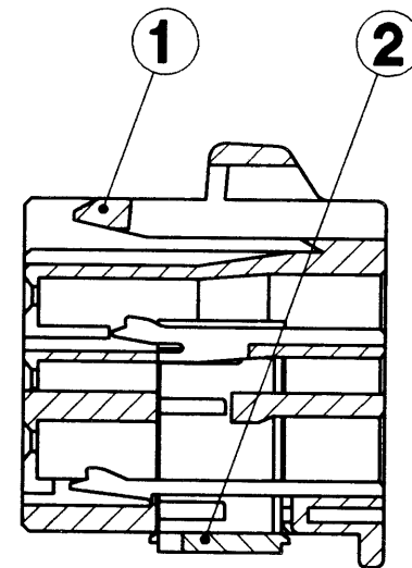
SEC. A-A
