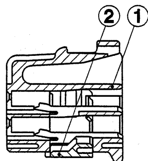
SEC. A-A
