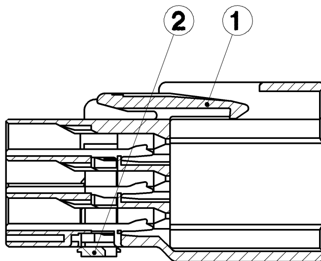
SEC. A-A
