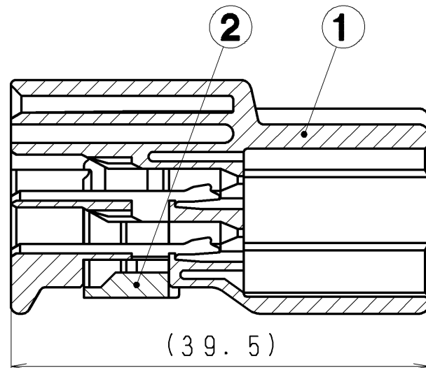
SEC. A-A
