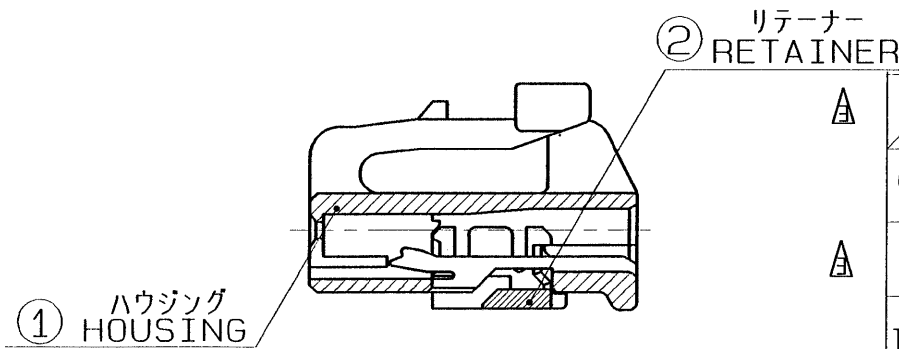
SEC. A-A
