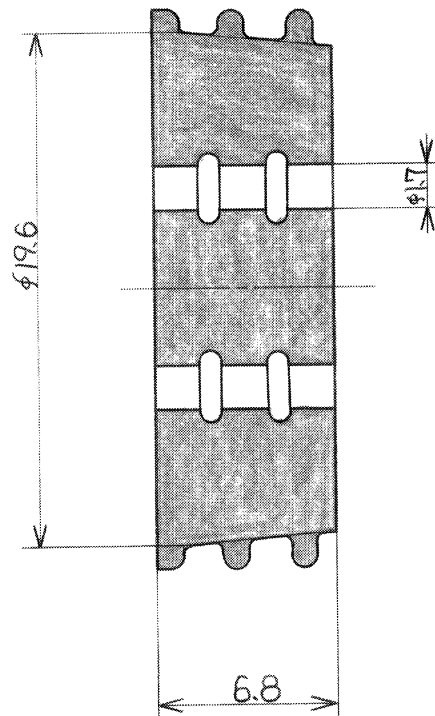
A-A 断面図
