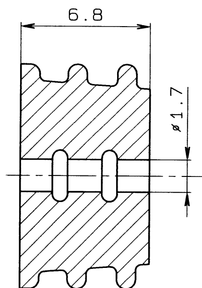
SEC. A-A
