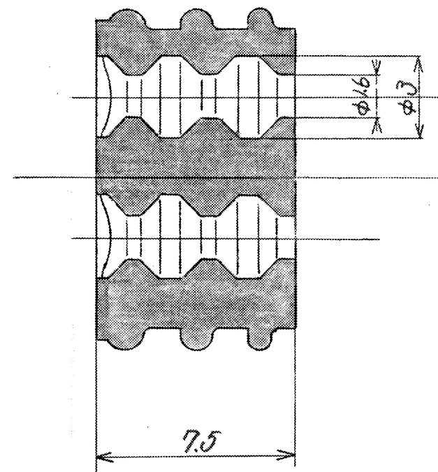
断面A-A
