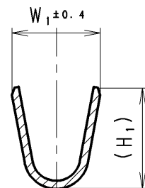
SEC. A-A
