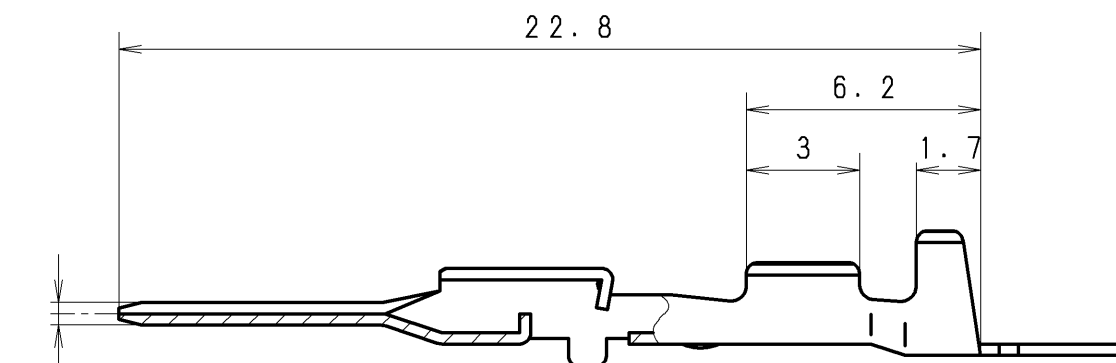
SECTION A-A
