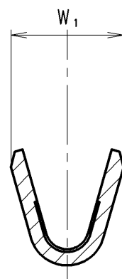
ワイヤーバレル (10:1) WIRE BARREL
