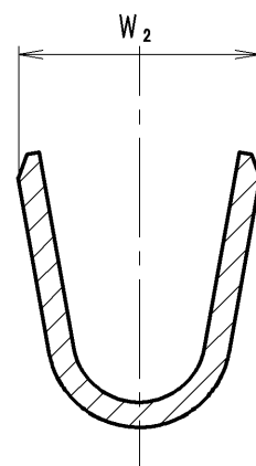
インシュレーションバレル (10 : 1) INSULATION BARREL
