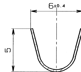
SEC. A-A
