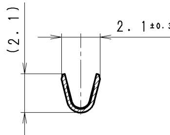
SEC. A-A
