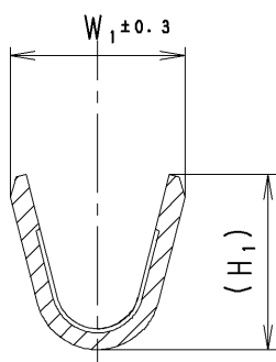
SEC. A-A
