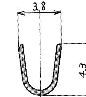
断面 AA
