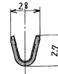
断面 BB
