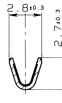
SEC. A-A
