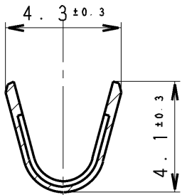
SEC. A-A
