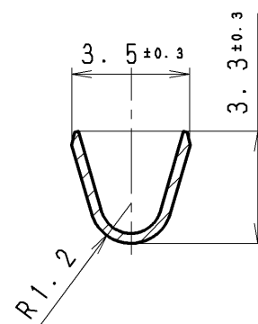
SEC. A-A
