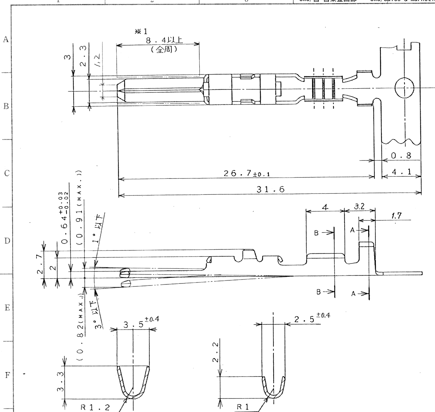
断面 B-B
