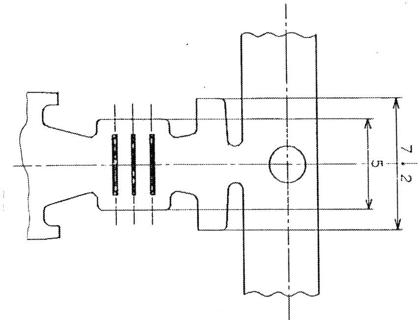
バレル部展開図
