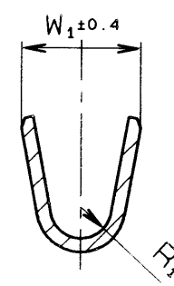
SEC. A-A
