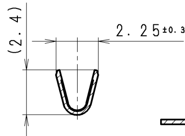
SEC. A-A
