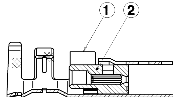
SEC. A- A
